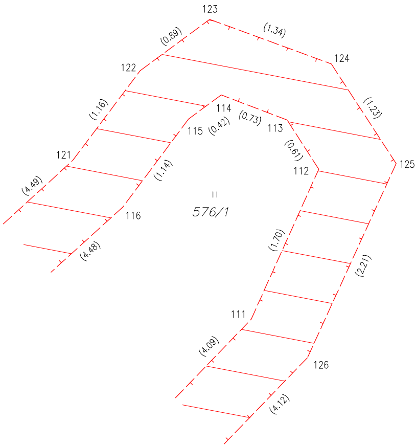
Detail:B
